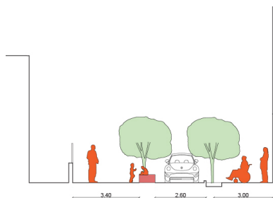
fig. 16 : Sección sin aparcamientos
